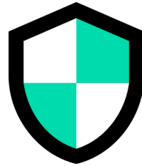
보안 취약
